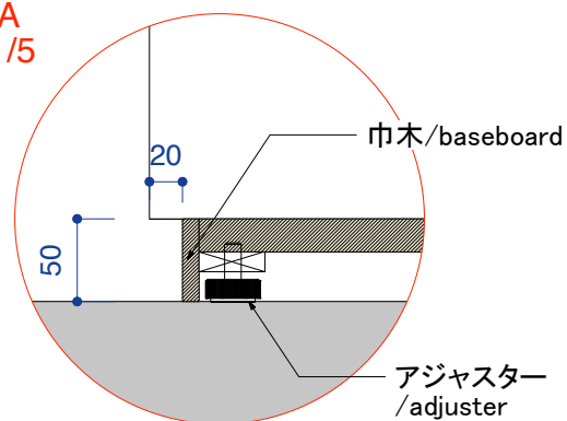
Detail-B scale:1/5
